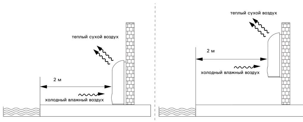
Схема установки
