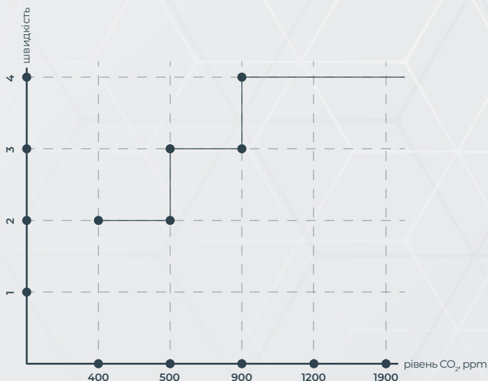
Графік роботи в автоматичному режимі (при наявності датчика CO₂)
